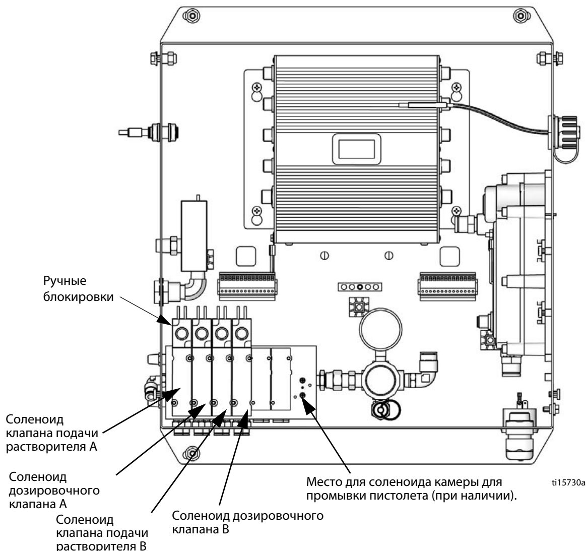
Рис. 19. Соленоидные клапаны в блоке управления
